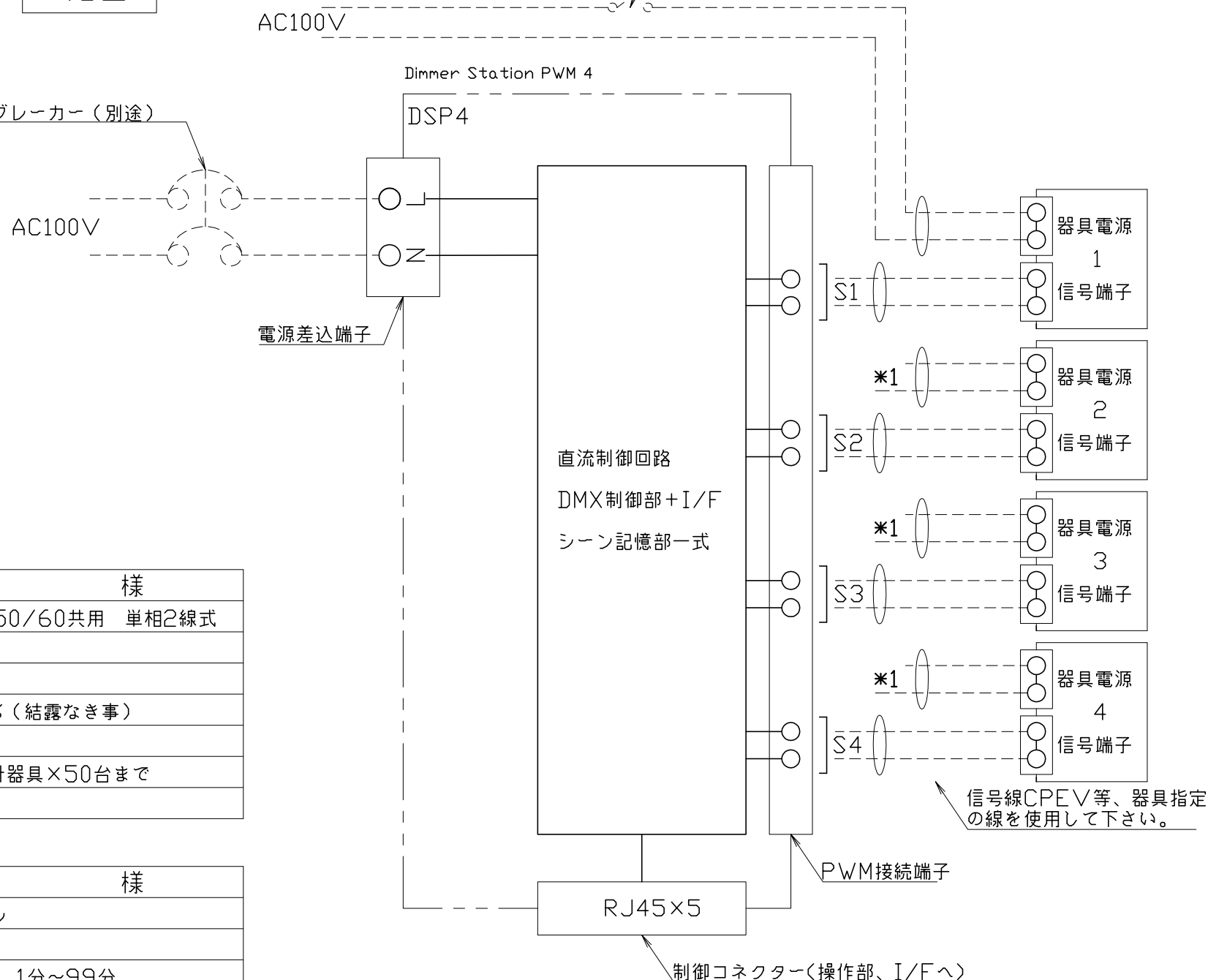
回路図
