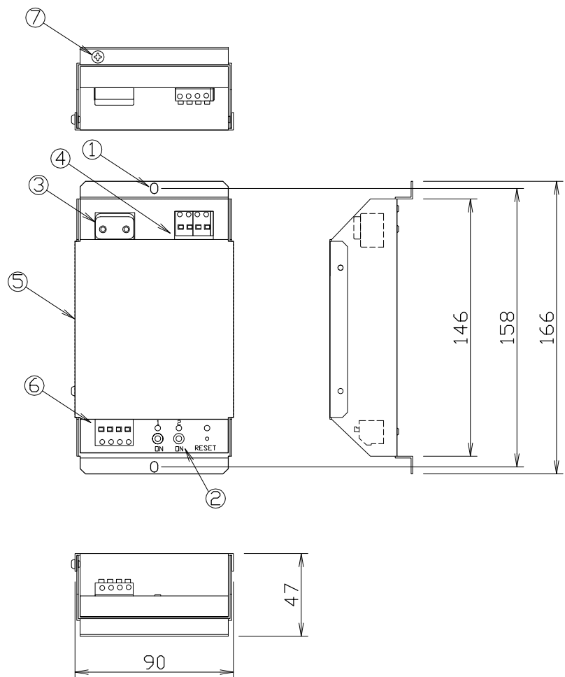
外形図
