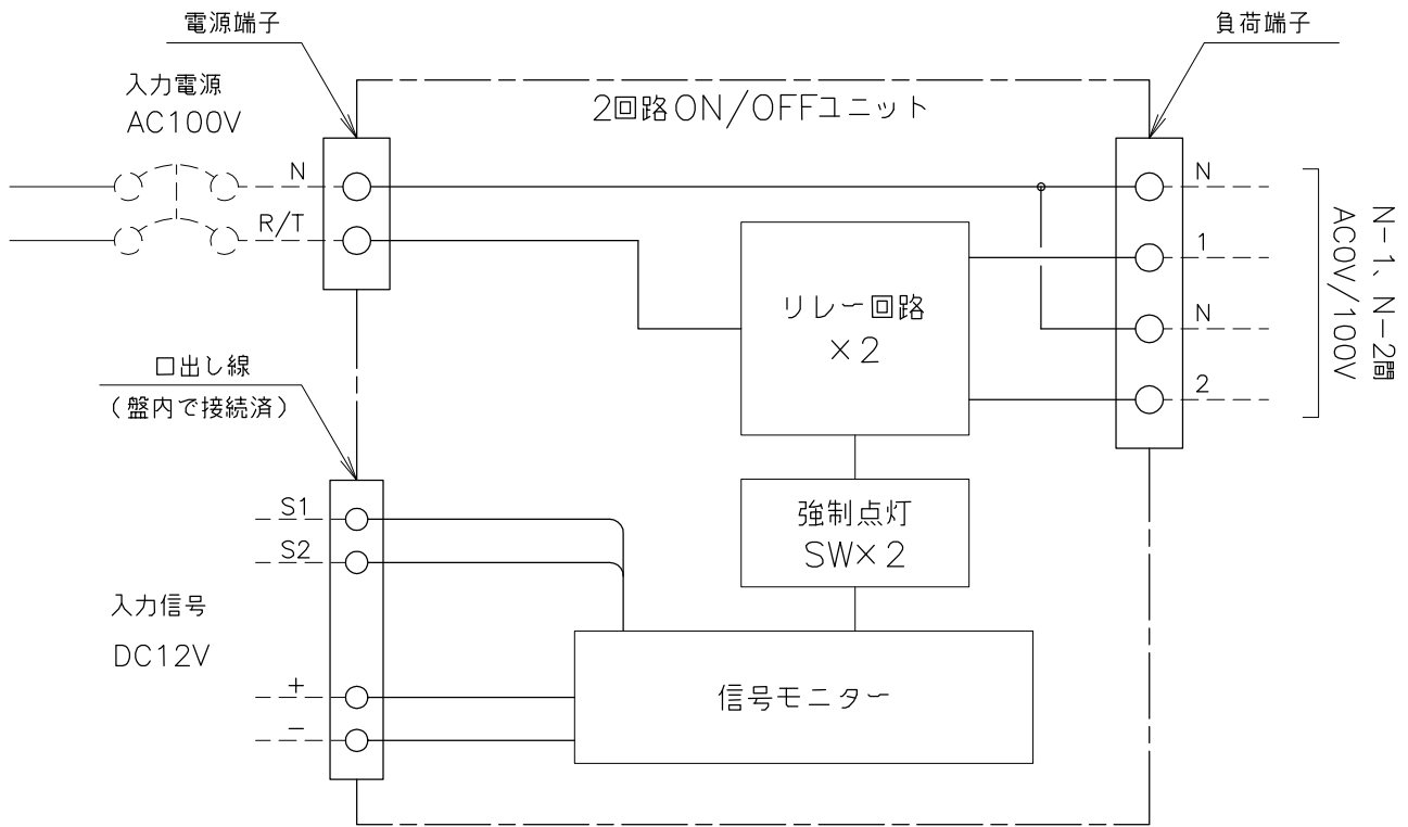
回路図
