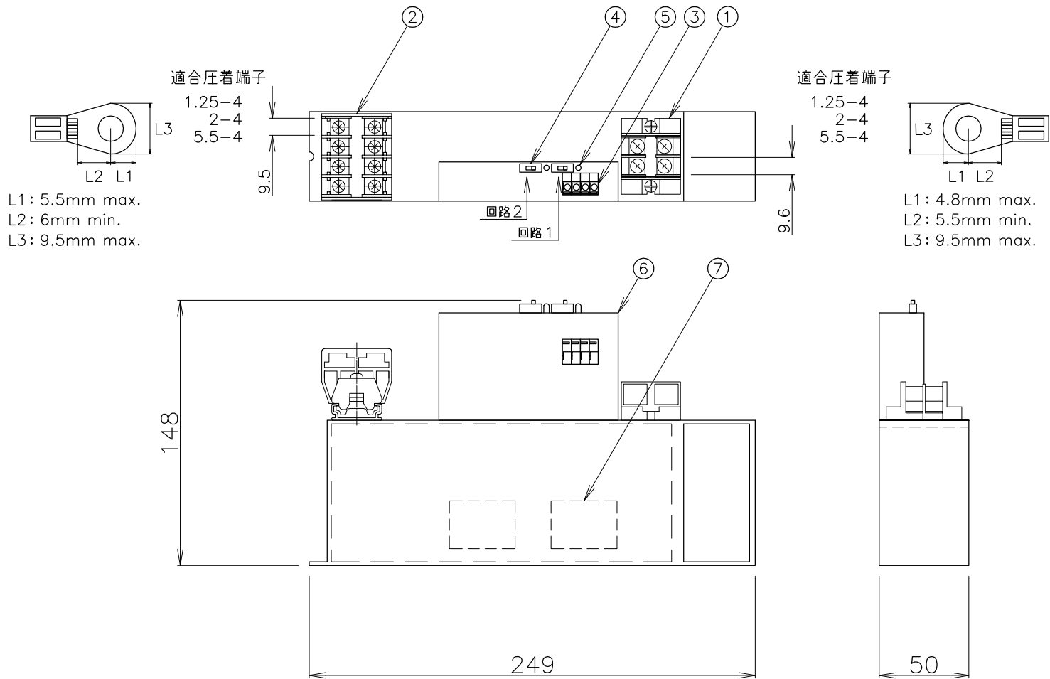
外形図
