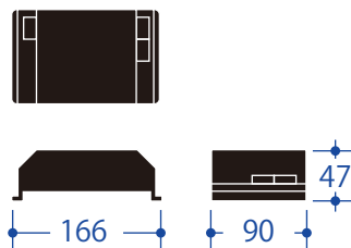
外形寸法
