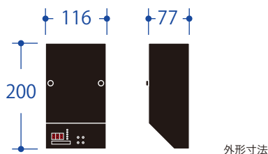
外形寸法
